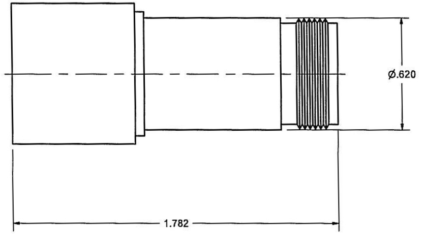
TYPE N SCALE 3 : 1
